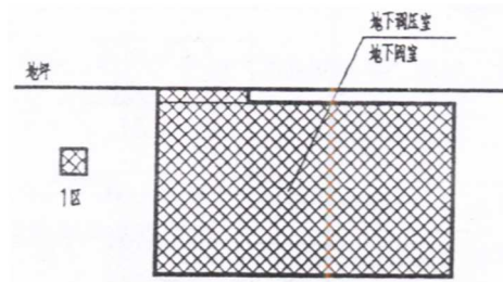
图 D-6 地下调压和地下阀室的爆炸危险区域等级和范围的划分
