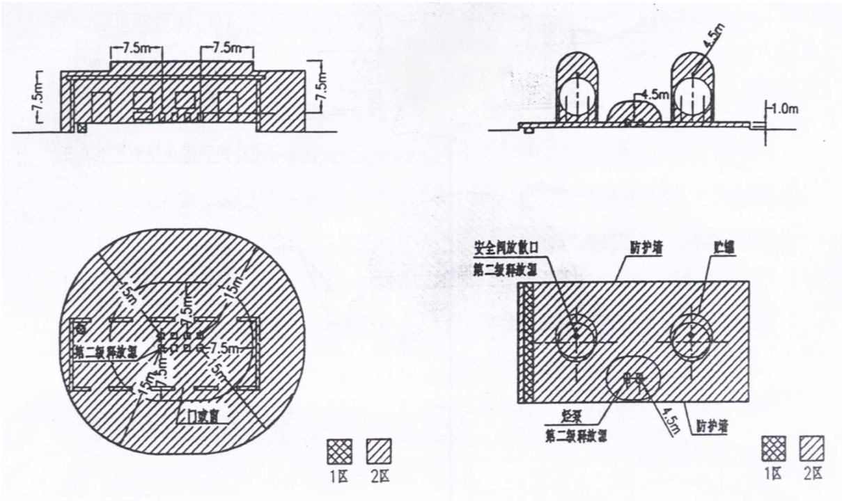
图 E.0.2 通风良好的生产性建筑爆炸危险区域等级和范围的划分
