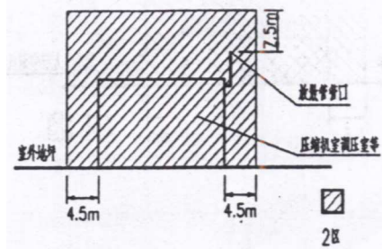
图 D-4 通风良好的压缩机室、调压室、计量室等生产用房的爆炸危险区域等级和范围的划分
