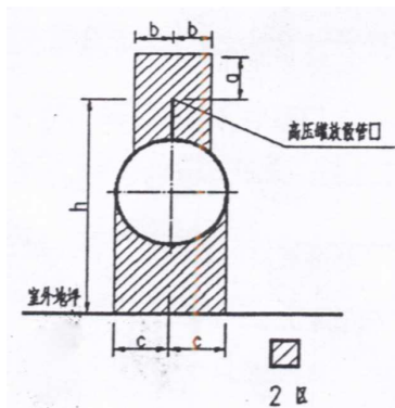
图 D-1 露天设置的固定容积储气罐的爆炸危险区域等级和范围的划分
