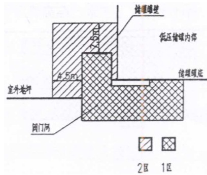
图 D-3 低压储气罐进出气管阀门间的爆炸危险区域等级和范围的划分
