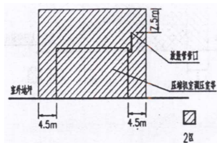
图 D-7 城市无人值守的燃气调压室的爆炸危险区域等级和范围的划分
