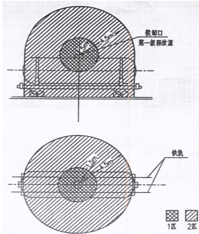
图 E.0.4 槽车装卸口处爆炸危险等级和范围的划分
