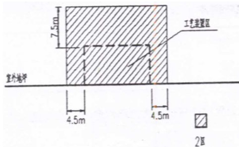
图 D-5 露天设置的工艺装置区的爆炸危险区域等级和范围的划分
