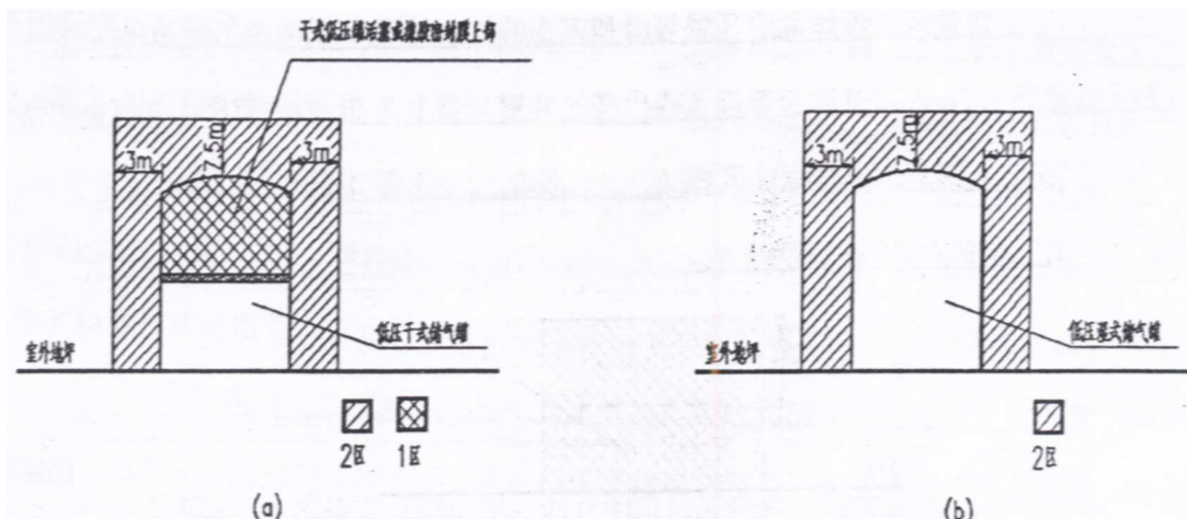
图 D-2 露天设置的低压储气罐的爆炸危险区域等级和范围的划分
